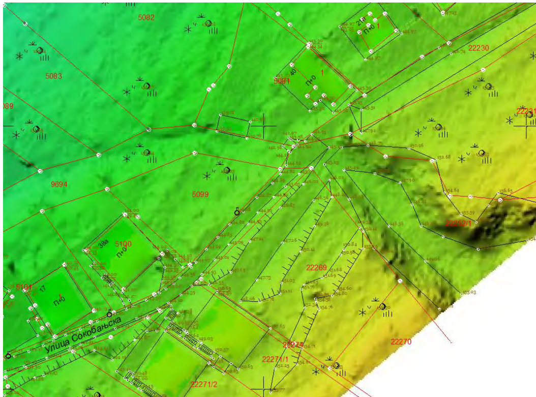
Слика 11: Интегрисана геореференцирана слика ДМТ
