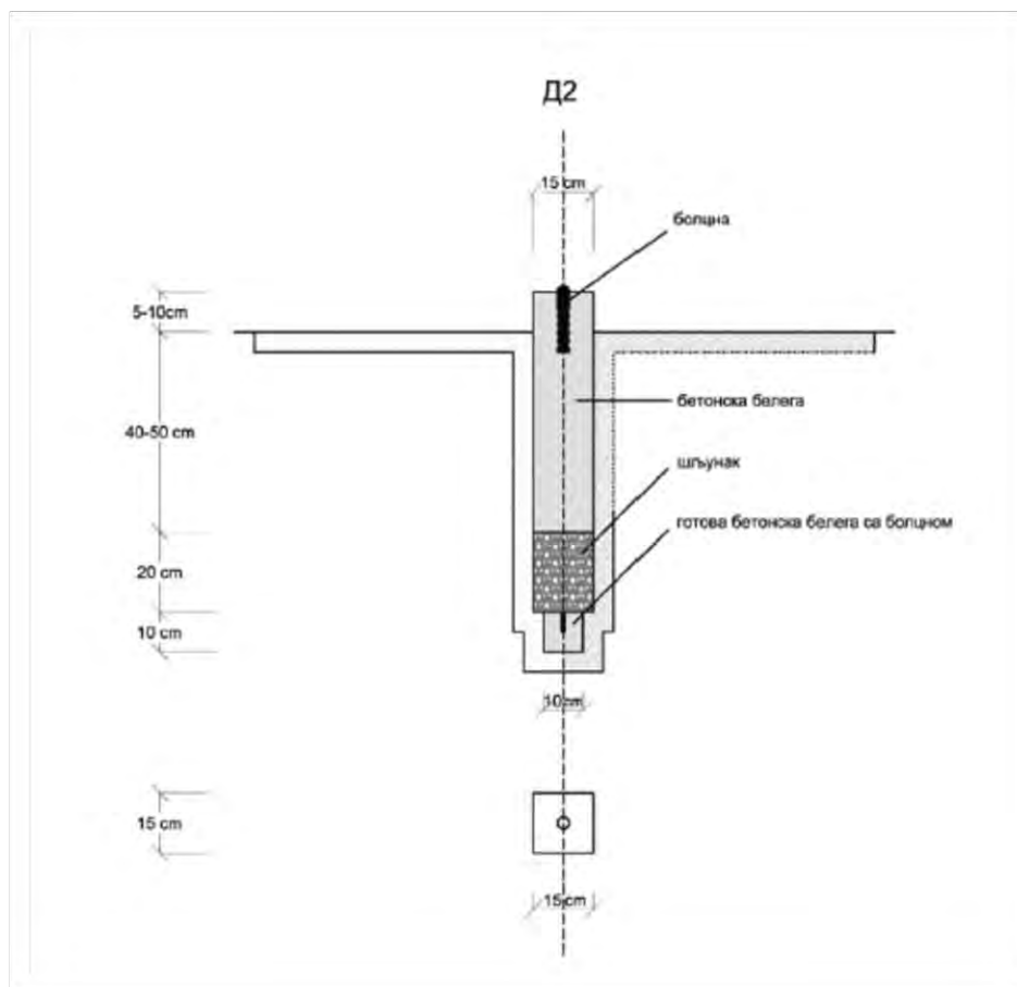
Слика 18: Изглед и димензије белеге ТИП Д2 са подземним центром
